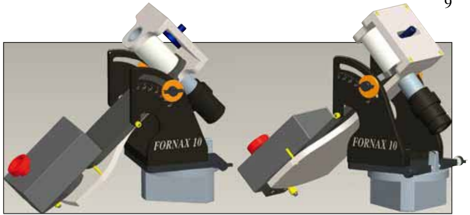
Abb. 6: Aufbau der Fornax-10-Montierung als Computergrafik [7]
