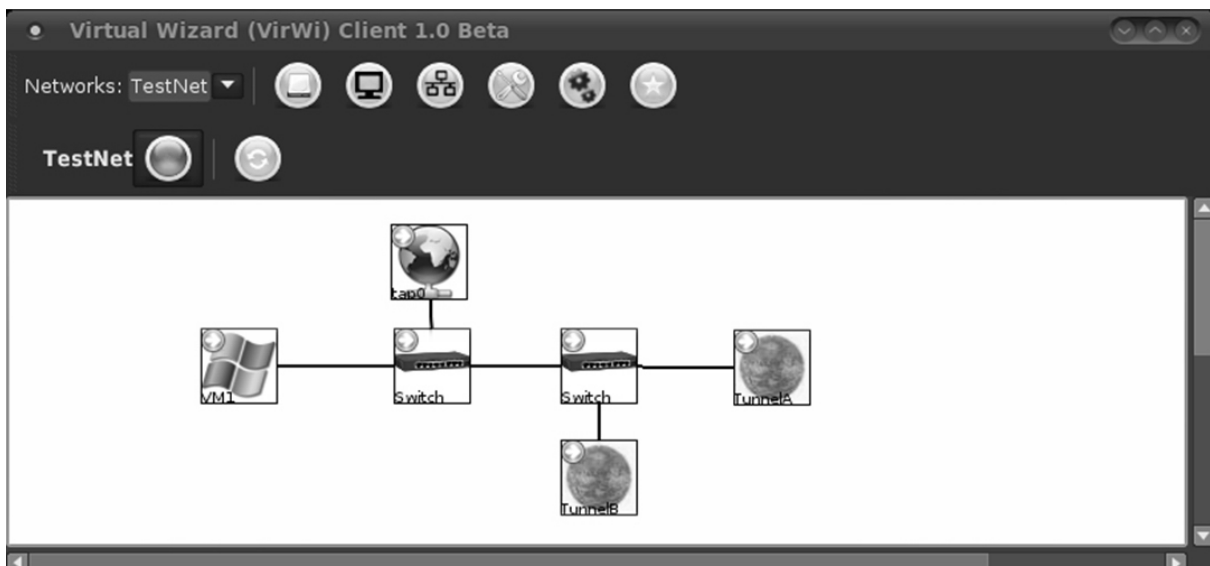
Abb. 1: VirWi-GUI
